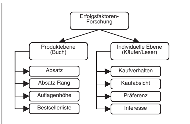
Abbildung 2: Überblick Erfolgsfaktorenforschung
