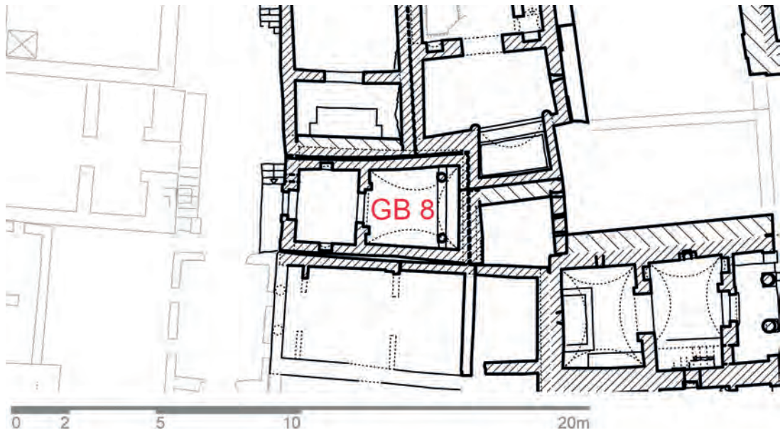
Abb. 2: Grundriss; 2021
