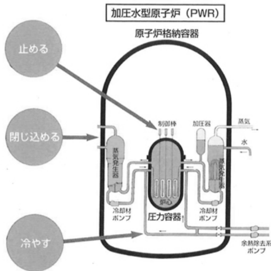
Abbildung 20: Das Bild soll den Mehrebenenenschutz darstellen. In den Kreisen links steht: „stoppen, eindämmen, kühlen“. Es stammt von der Homepage des Ikata Atomkraft-PR-Zentrums ( http://www.pikara.ne.jp/dr-sada/know/index10.html ).
