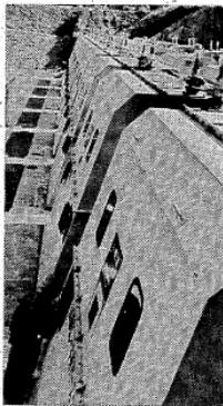
東海第二自備のクワゲ対策機。クワゲリレー中、ロータリースクリーンが各台必ずある。
