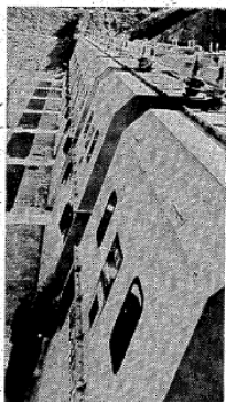
東海第二原子力発電所のクラゲ対策施設、ローケリール、ローケリールスクリーンが各5台ずつある
