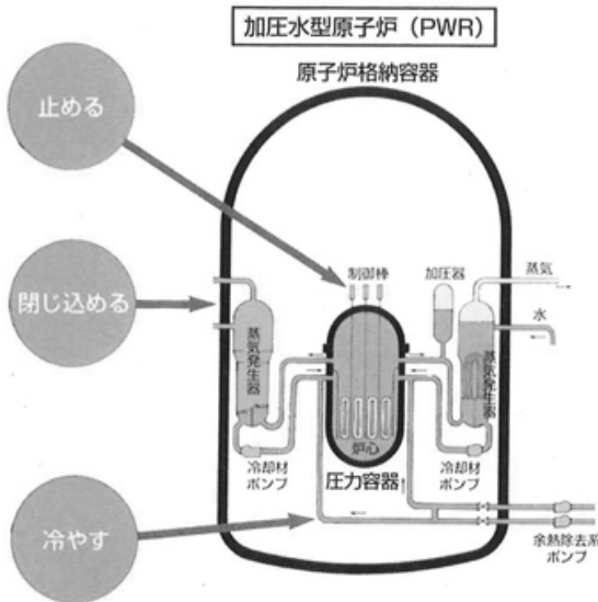
Abbildung 20: Das Bild soll den Mehrerebenen-Schutz darstellen. In den Kreisen links steht: „stoppen, eindämmen, kühlen“. Es stammt von der Homepage des Ikata Atomkraft-PR-Zentrums ( http://www.pikara.ne.jp/dr-sada/known/index10.html ).
