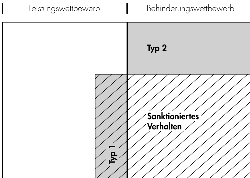
Grafik 5: Fehler erster und zweiter Ordnung
