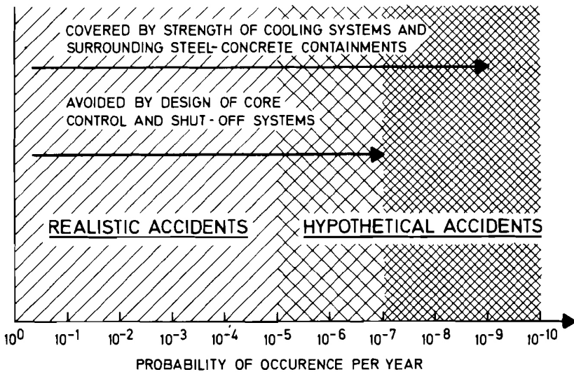
Abb. 1: Matrix möglicher Unfälle zwischen realistischen und hypothetischen Szenarien und Typen von Sicherheitsmaßnahmen
