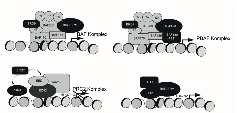
Abbildung 2: Beispiele für das Zusammenspiel verschiedener Proteine in Chromatinkomplexen und die Auswirkung auf die Gentranskription
