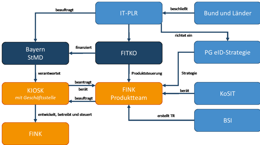
Abbildung 3: Organisationsstruktur KIOSK
