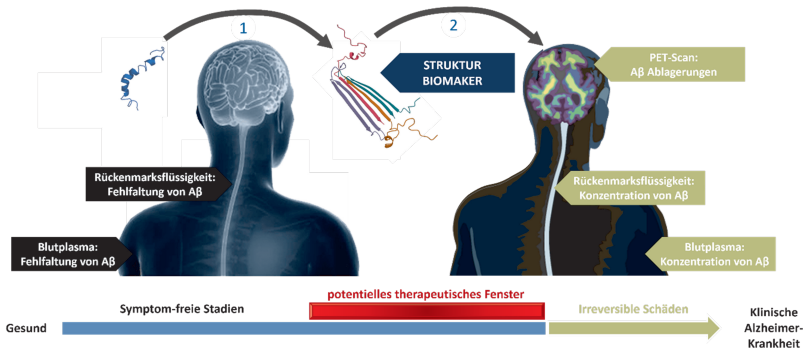
Abbildung 1: Die Umfaltung des A \beta -Peptids von einer \alpha -helikalen bis ungeordneten Struktur (blau, 1) hin zu \beta -Faltblatt-Sekundärstrukturen (bunt) ist der initiale Schritt in der Entstehung von Alzheimer und führt im weiteren Verlauf zu neurotoxischen Ablagerungen, den sogenannten Plaques, im Gehirn (2). Diese können dann mittels PET-Scan sichtbar gemacht werden.
