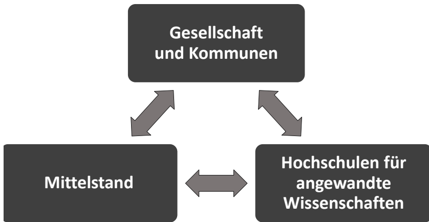
Abbildung 2: Regionale Innovationsökosysteme
