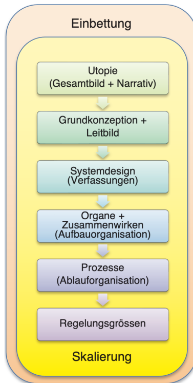
Abbildung 21: Achteiliger Modellbildungs-Prozess
