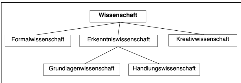
Abbildung 3: Ergänzte Wissenschaftssystematik 14
