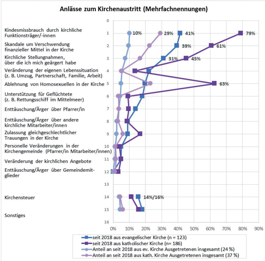
Abbildung 4: Austrittsanlässe
