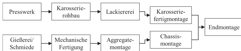
Abbildung 2: Prozesskette der Gewerke bei der Automobilproduktion
