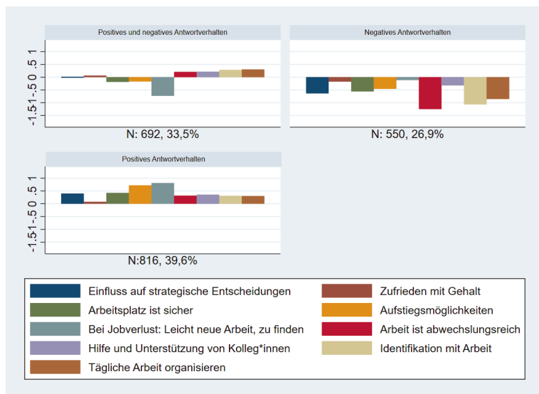
Abbildung 3: Drei-Clusterlösung
