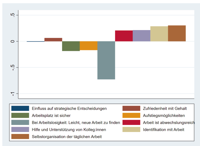
Abbildung 5: Cluster 2
