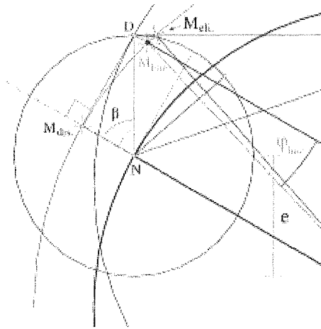
Abb. 23: Pausbäckige und elliptische Bahnkonstruktion
