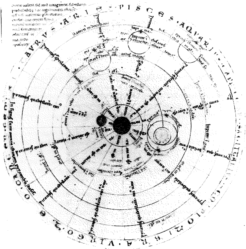
Abb. 6: K benhavn Kongelige Bibliotek ms. G.K.S. 277. fol., f. 49r (1254?): Capella-Modell integriert in eine epizyklische Planetentheorie.
