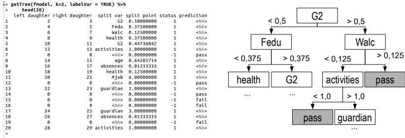
Abbildung 7.2: Die ersten 20 Einträge eines Baumes in einem Random Forest in Tabellen- und Baumform, Quelle: eigene Darstellung.
