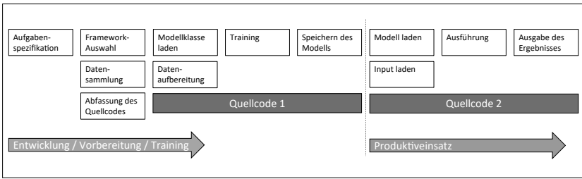
Abbildung 6.2: Entstehung eines ML-Modells, vereinfachte, eigene Darstellung.
