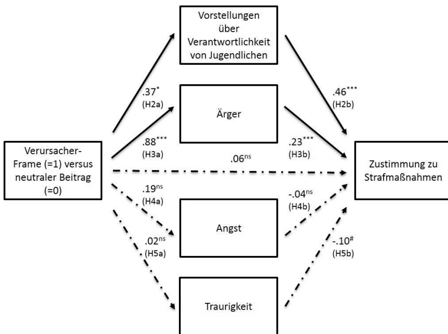
Abbildung 2: Multiples Mediationsmodell
